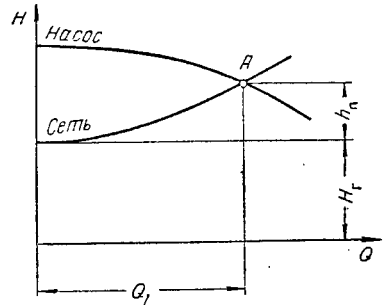
Рис. III-8. Совмещение характери- стик насоса и сети.
