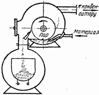
Рис. XV-32. Одновальцовая сушилка.
