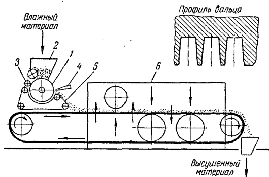
Рис. XV-33. Одновальцовая формующая сушилка:
