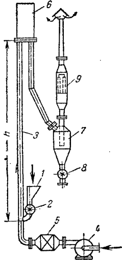
Рис. XV-28. Пневматическая сушилка:
