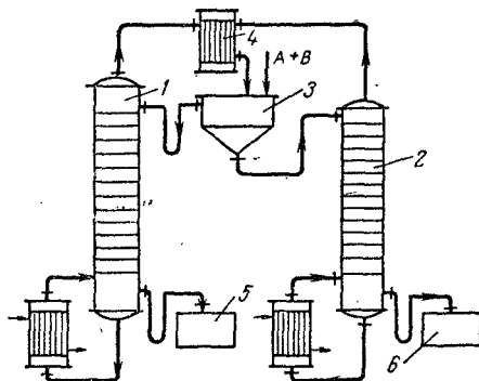
Рис. XII-33. Схема двухколонной установки для гетероазеотропной ректификации бинарных расслаивающихся жидкостей:
