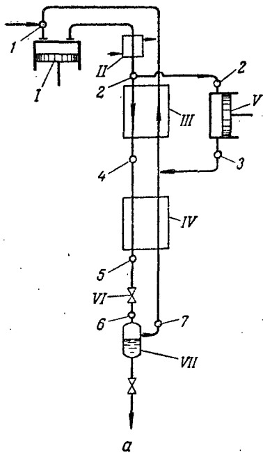
Рис. XVII-17. Соединенные циклы дроссельный и детандерный без регенерации: а — принципиальная схема установки; б — изображение процесса на диаграмме T-S ; 1 — компрессор; II — холодильный компрессор; III — регенеративный теплообменник, в котором используется холод детандерного цикла; IV — регенеративный теплообменник; V — детандер; VI — дроссель; VII — сборник жидкого продукта.
