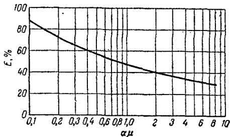
Рис. XII-25. График для определения средней эффективности колонны E в зависимости от произведения летучести компонентов \alpha на среднюю молярную вязкость жидкости питания \mu (в снз ).
