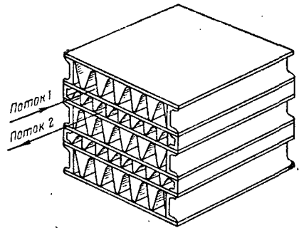
Рис. VIII-23. Схема устройства пластинчато-ребристого теплообменника. Поток 1, Поток 2.
