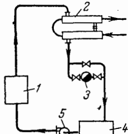
Рис. VIII-1. Схема нагрева глухим паром:
