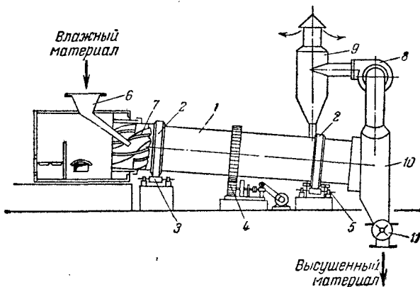
Рис. XV-22. Барабанная сушилка:
