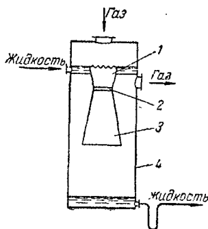
Рис. XI-29. Распыливающий абсорбер Вентури:
