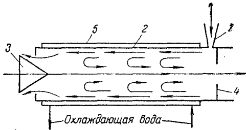
Рис. XVII-4. Вихревая труба:
