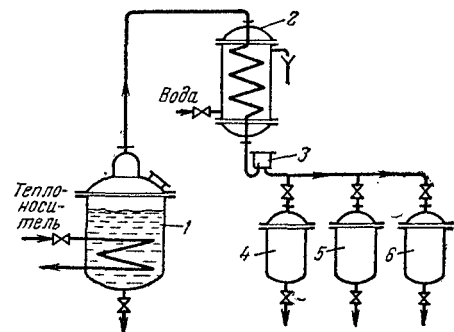
Рис. XII-8. Схема установки для фракционной перегонки:
