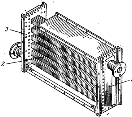
Рис. VIII-22. Пластинчатый калорифер: 1 — коллектор для входа пара; 2 — оребренная труба; 3 — коллектор для приема конденсата.
