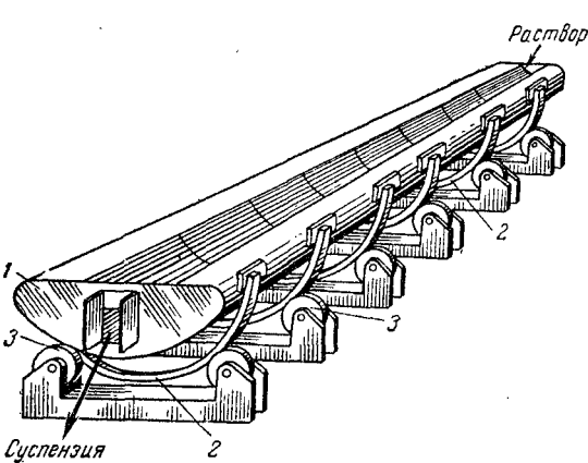
Рис. XVI-6. Качающийся кристаллизатор: 1 — корыто; 2 — бандаж; 3 — опорные ролики.
