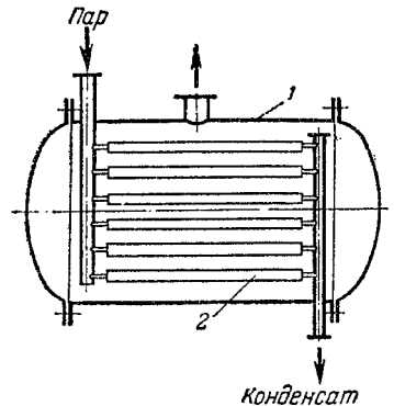
Рис. XV-29. Вакуум-сушильный шкаф:
