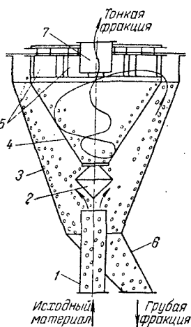
Рис. XIX-8. Схема воздушно-проходного сепаратора:
