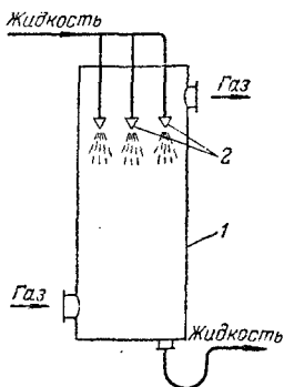
Рис. XI-28. Полая распыливающий абсорбер:
