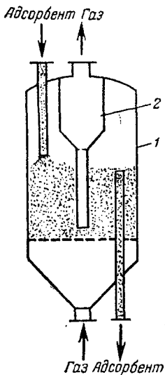
Рис. XIV-8. Однокамерный адсорбер с кипящим слоем поглотителя:
